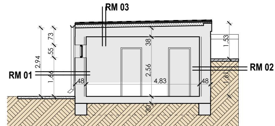
C-C METSZET
