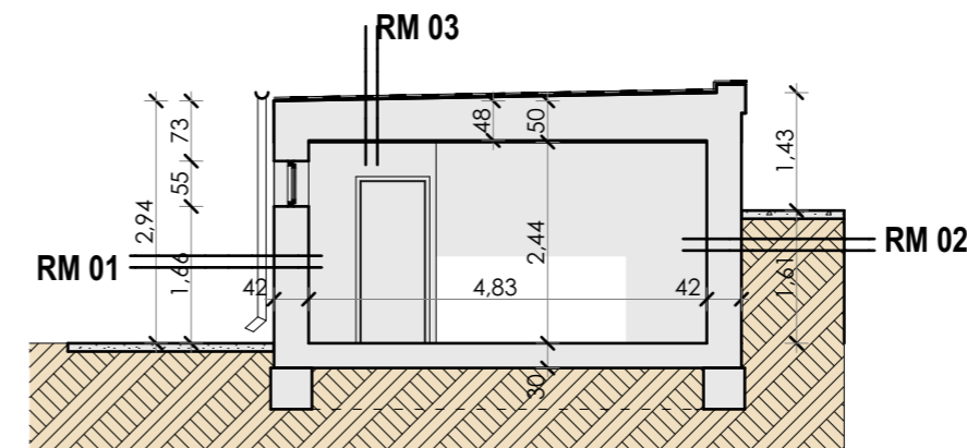
B-B METSZET
